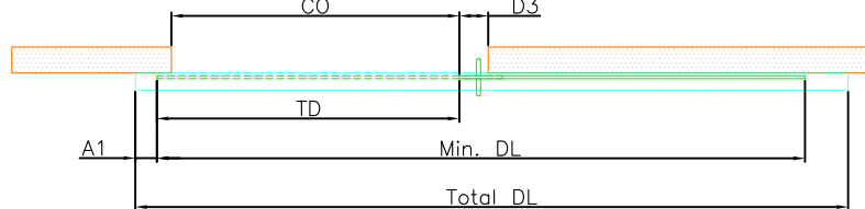
SECTION B-B DOOR OPEN
