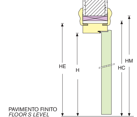
SEZIONE VERTICALE VERTICAL CROSS-SECTION
