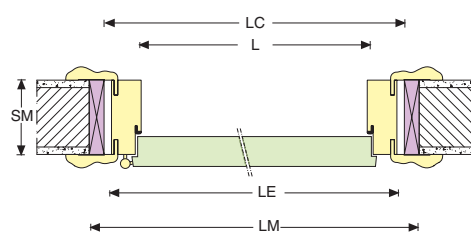
SEZIONE VERTICALE VERTICAL CROSS-SECTION
