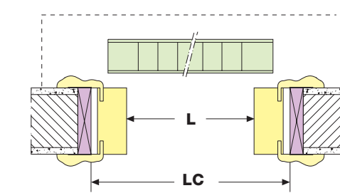
SEZIONE ORIZZONTALE HORIZONTAL CROSS-SECTION
