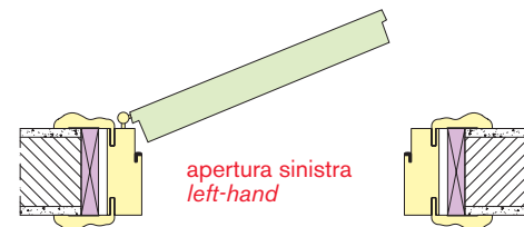
SEZIONE ORIZZONTALE HORIZONTAL CROSS-SECTION
