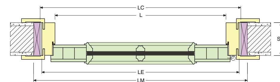
SEZIONE ORIZZONTALE HORIZONTAL CROSS-SECTION
