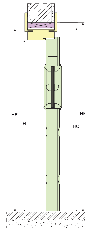
SEZIONE VERTICALE VERTICAL CROSS-SECTION
