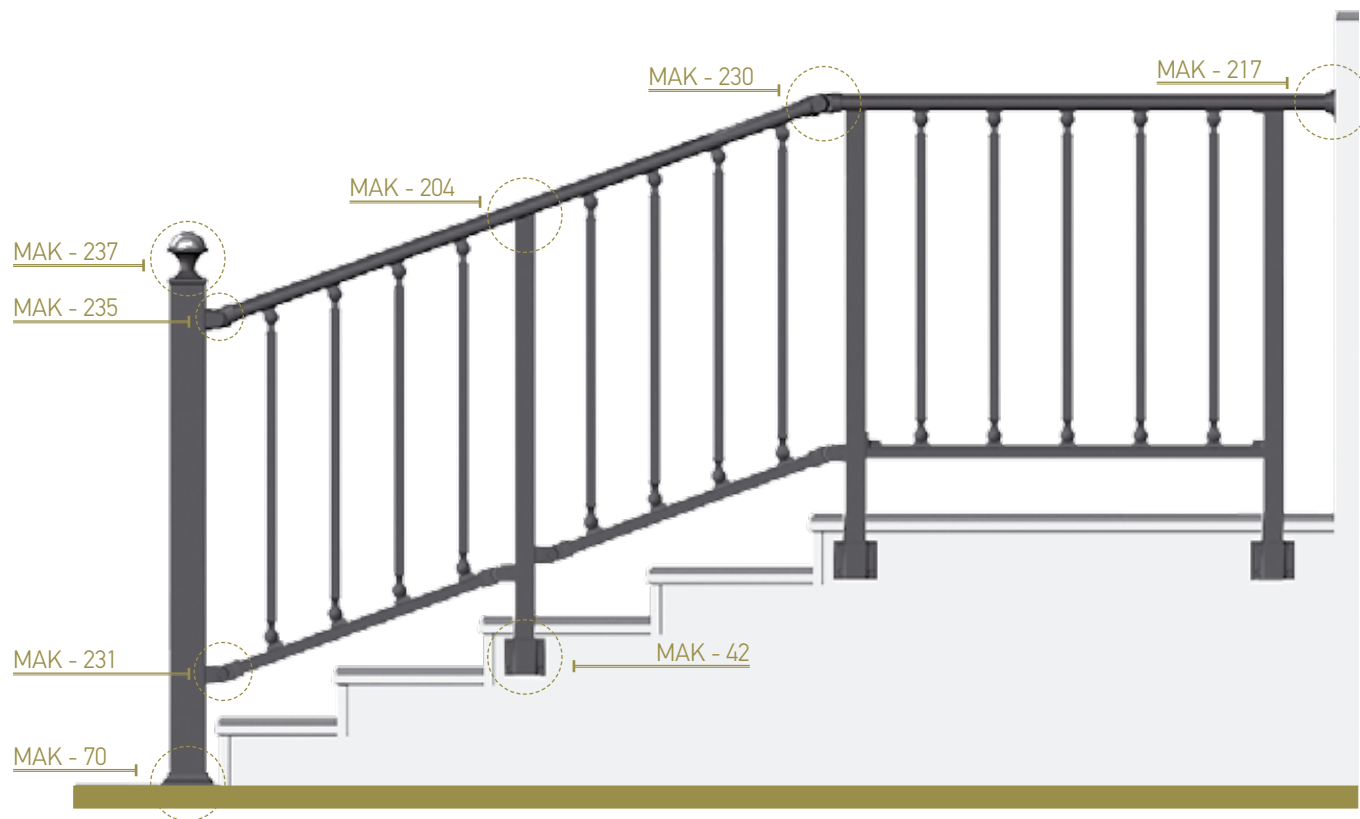
external rail support for narrow stairs, with column MAK - 140 and MAK - 42 base support extérieur de garde - corps pour escaliers avec colonne MAK - 140 et base MAK - 42
