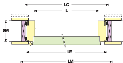
SEZIONE VERTICALE VERTICAL CROSS-SECTION
