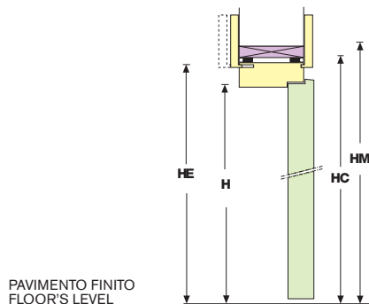
SEZIONE VERTICALE VERTICAL CROSS-SECTION
