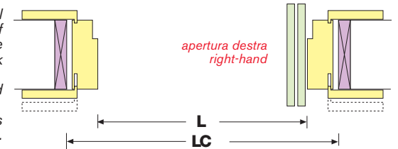
SEZIONE VERTICALE VERTICAL CROSS-SECTION
