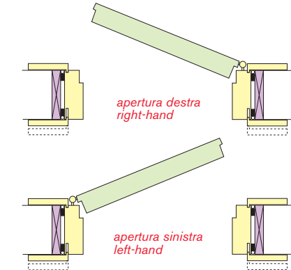
SEZIONE ORIZZONTALE HORIZONTAL CROSS-SECTION
