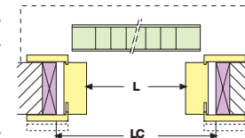
SEZIONE ORIZZONTALE HORIZONTAL CROSS-SECTION
