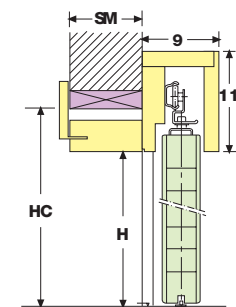
SEZIONE VERTICALE VERTICAL CROSS-SECTION
